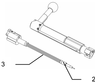
Démontage du percuteur
