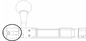
Attelage de percuteur en position d'insertion
