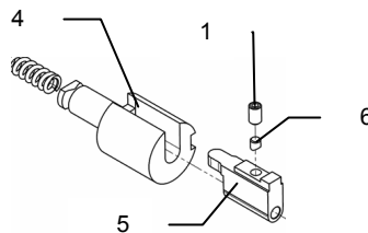
Démontage du percuteur
