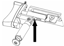
Réglage de la longueur
